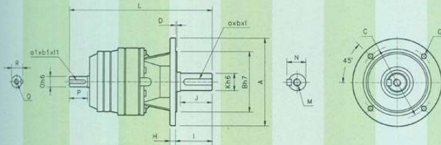
尺寸規格表 DIM.TABLE(mm)
